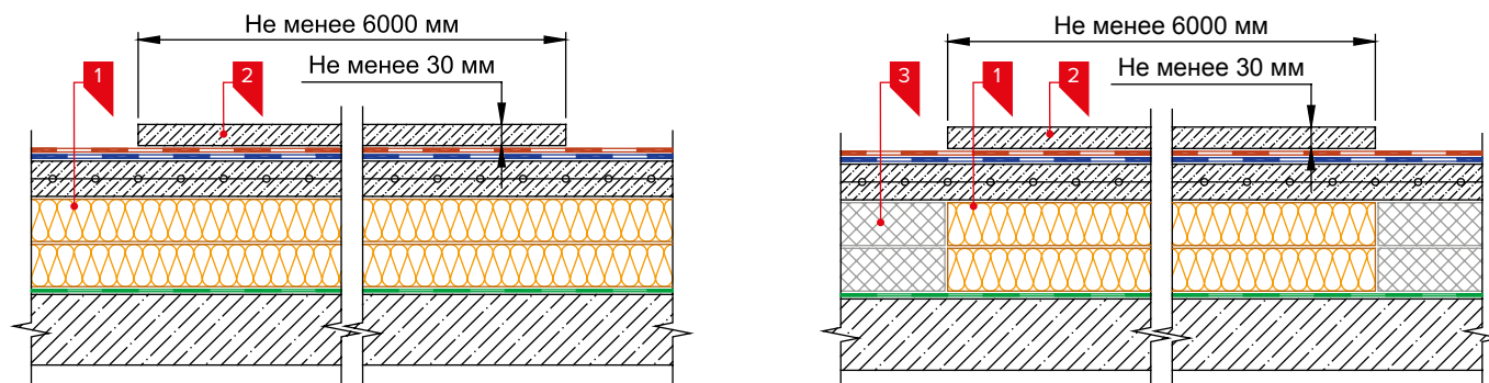
Рис. 4.1. Варианты устройства противопожарных рассечек 1. Утеплитель НГ и Г1; 2. Монолитная стяжка; 3. Утеплитель Г3-Г4
