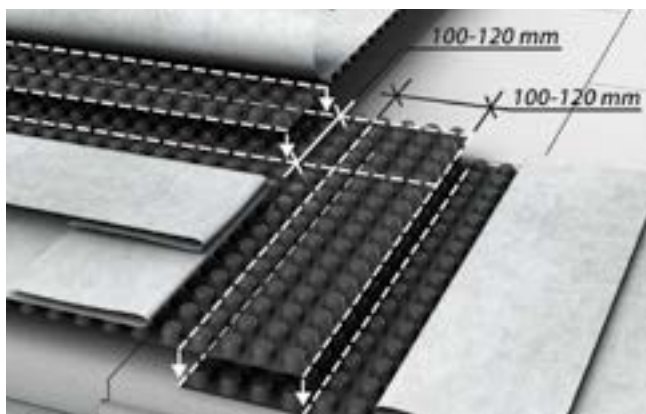
Рис. 3.50. Устройство нахлестов дренажной мембраны
