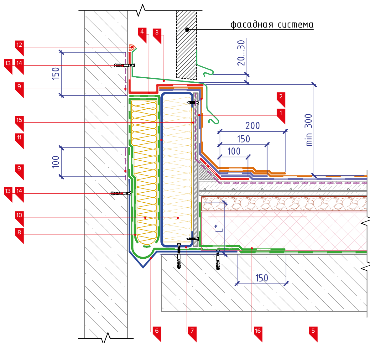
Рис. 3.60. Тип Д. Деформационный шов в месте сопряжения двух разновысоких частей здания
