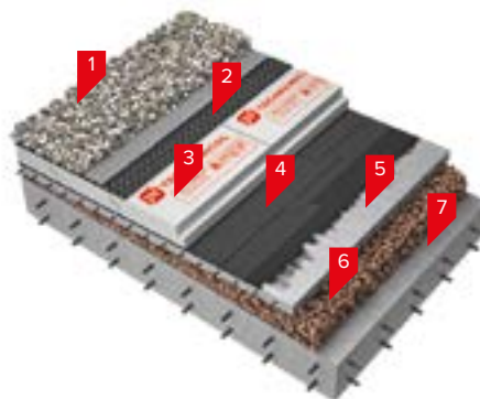
Рис. 1.2. Конструкция инверсионной крыши
