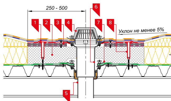
Рис. 3.51б. Примыкание к двухуровневой воронке 1. слой усиления – Техноэласт ЭПП; 2. экструзионный пенополистирол ТЕХНОНИКОЛЬ CARBON PROF; 3. хризотилцементный пресованный плоский лист толщиной не менее 10 мм; 4. листоуловитель; 5. водоприемная воронка ТехноНИКОЛЬ; 6. надставной элемент; 7. обжимной фланец; 8. пластиковый элемент ТехноНИКОЛЬ
