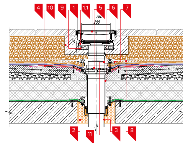
Рис. 3.52. Организация поверхностного водоотвода 1. лоток полимербетонный с вертикальным водоотводом; 1.1. решетка водоприемная щелевая чугунная; 2. заполнить монтажной пеной ТЕХНОНИКОЛЬ PROFESSIONAL 70; 3. водоприемная воронка ТЕХНОНИКОЛЬ; 4. дополнительный слой водоизоляционного ковра – Техноэласт ЭПП; 5. дренажное кольцо Д2; 6. надставной элемент воронки; 7. обжимной фланец; 8. геотекстиль иглопробермообработанный ТЕХНОНИКОЛЬ 300 г/м 2 ; 9. выравнивающий слой цементно-песчаный раствор М150; 10. бетонная обойма монолитный цементобетон В35; 11. надставной элемент водоприемной воронки
