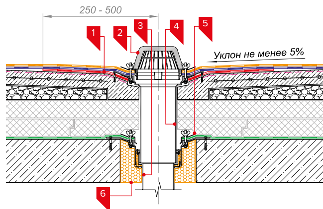
Рис. 3.51а. Примыкание к двухуровневой воронке 1. дополнительный слой водоизоляционного ковра – Техноэласт ЭПП; 2. листоуловитель; 3. водоприемная воронка ТЕХНОНИКОЛЬ; 4. надставной элемент с манжетой для водоприемной воронки ТЕХНОНИКОЛЬ; 5. обжимной фланец; 6. пена монтажная ТЕХНОНИКОЛЬ PROFESSIONAL 70
