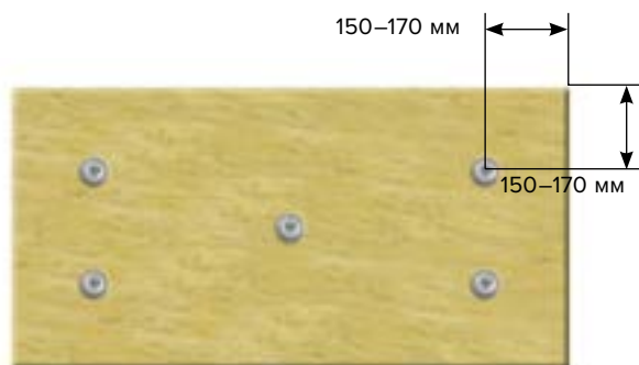
Рис. 4.2. Крепеж для крепления огнезащитных плит
