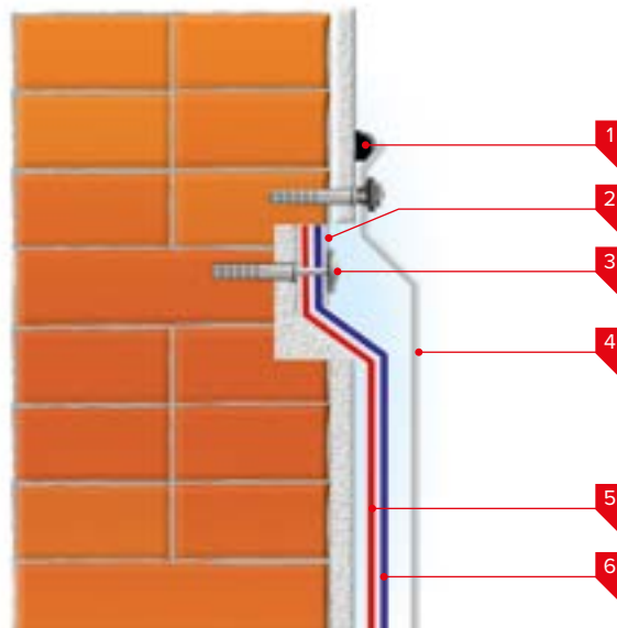
Рис. 3.26. Устройство широкой штробы
