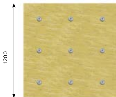
Рис. 4.3. Крепление огнезащитных плит к профлисту
